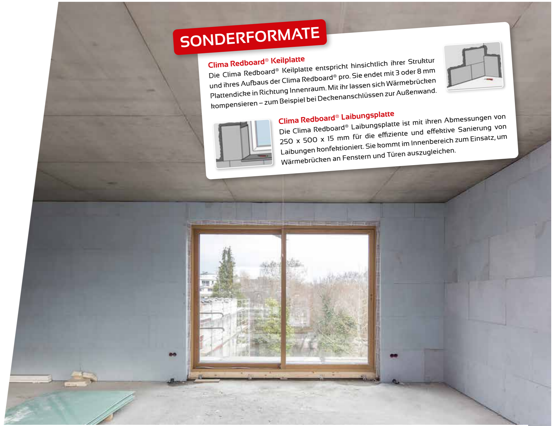
Altbauziegel mit Clima Redboard® pro in einer Dicke von 5 cm: U-Wert = 0,65 m 2 K/W
