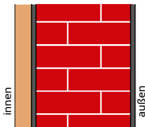
Altbauziegel mit Clima Redboard® pro in einer Dicke von 5 cm: U-Wert = 0,65 m 2 K/W
