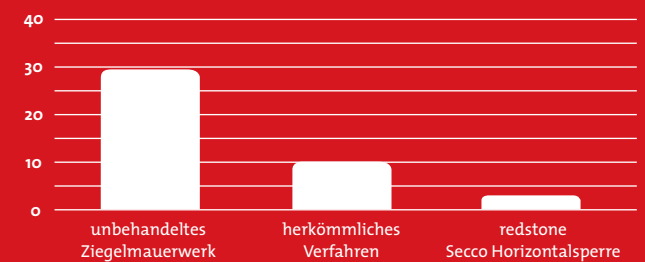
Kapillare Wasseraufnahme von Mauerwerk nach einer Woche (in %)
