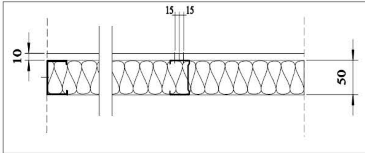
Abb.: Ausbildung einer Stoßfuge auf Metallständerkonstruktion
